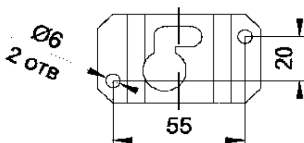
Рис.2.1 Координаты отверстий крепления кронштейна модуля.
