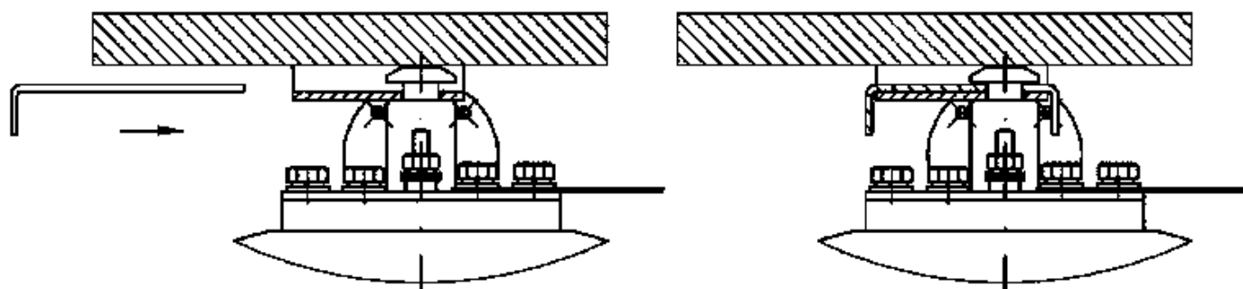
Рис.2.2 Схема крепления модуля.
