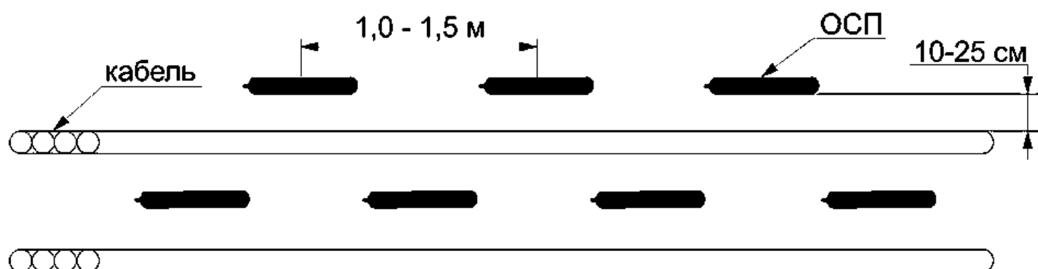
Рис. 3 Варианты размещения ОСП.
