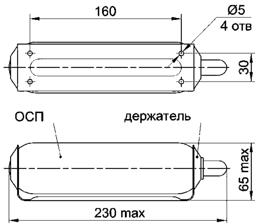
Рис. 2.1 ОСП с держателем защелка.
