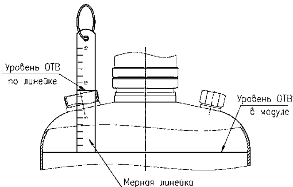
Рис.3. Измерение уровня ОТВ.
