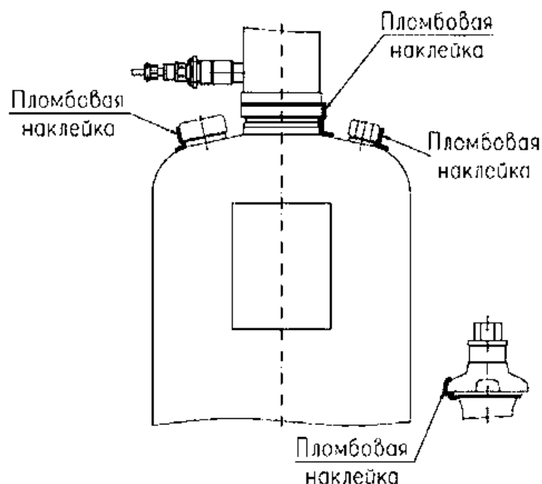
Рис.4. Места установки пломбовых наклеек.
