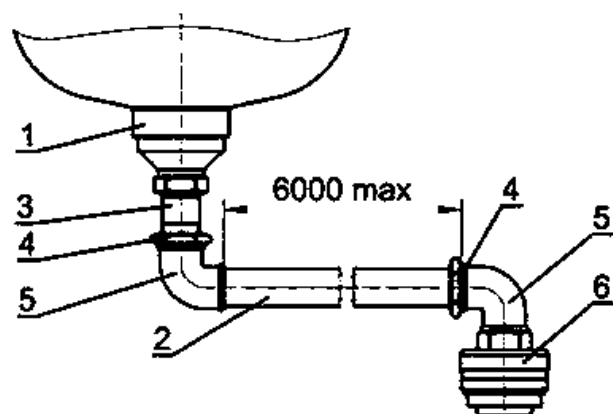
Рис.7. Монтажная схема распределительного трубопровода для модификаций «Буран-15TPBTHT6», «Буран-15TPBTHT4».
