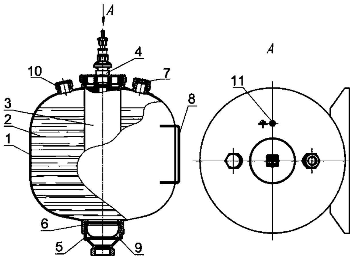
Рис.6. Устройство модуля пожаротушения тонкораспыленной водой «Буран-15ТРВТНТ».
