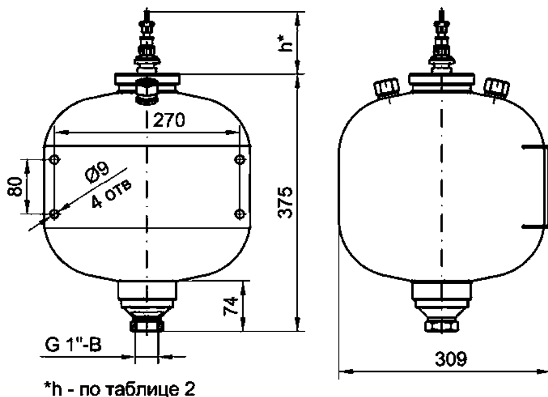
Рис. 1. Габаритные и присоединительные размеры модификаций модулей пожаротушения тонкораспылённой водой «Буря-15ТРВТНТ».
