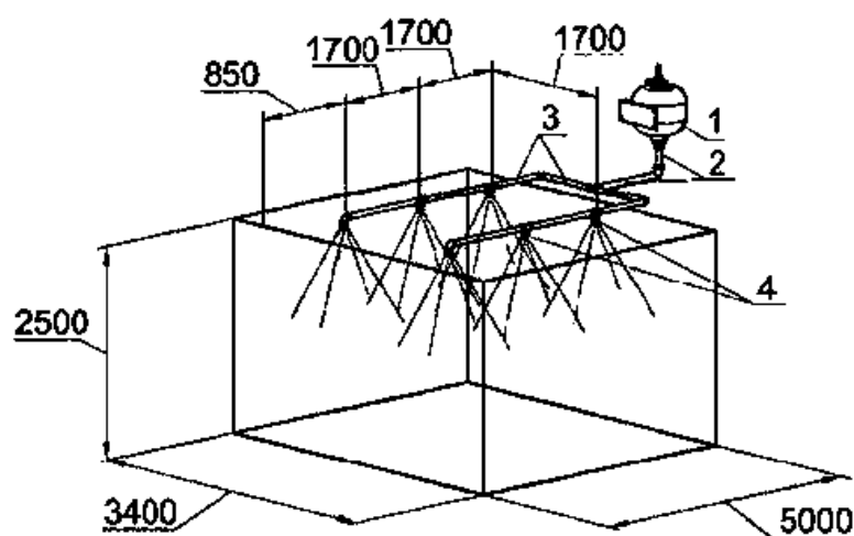
Рис.9. Монтажная схема распределительного трубопровода для модуля «Буран-15TPBTHT2,5», состоящего из двух ветвей.
