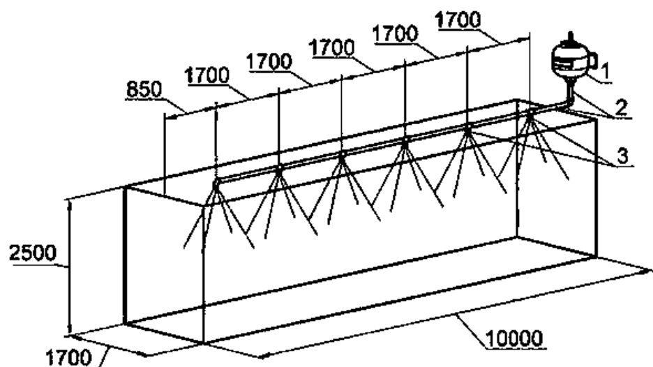
Рис.10. Монтажная схема распределительного трубопровода для модуля «Буран-15TPBTH2,5», состоящего из одной ветви.
