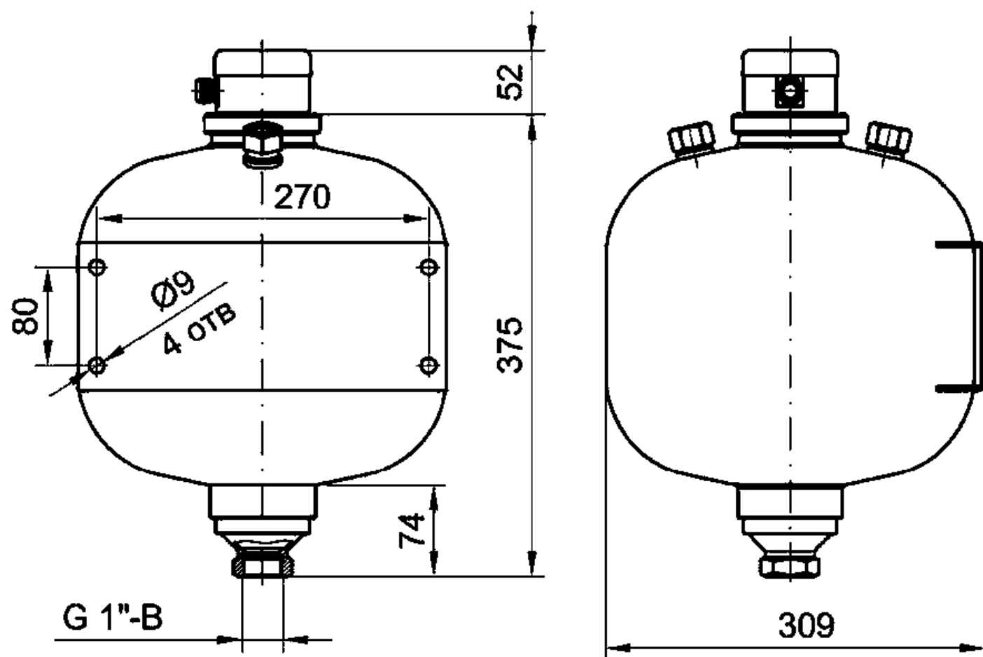
Рис. 1. Габаритные и присоединительные размеры модификаций модулей пожаротушения тонкораспыленной водой «Буря-15ТРВТНТ(У1)».
