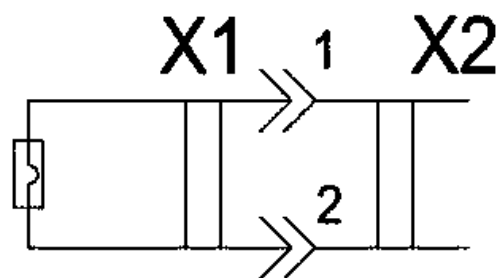
Рис.11. Электрическая схема подключения модуля к шлейфу пуска
