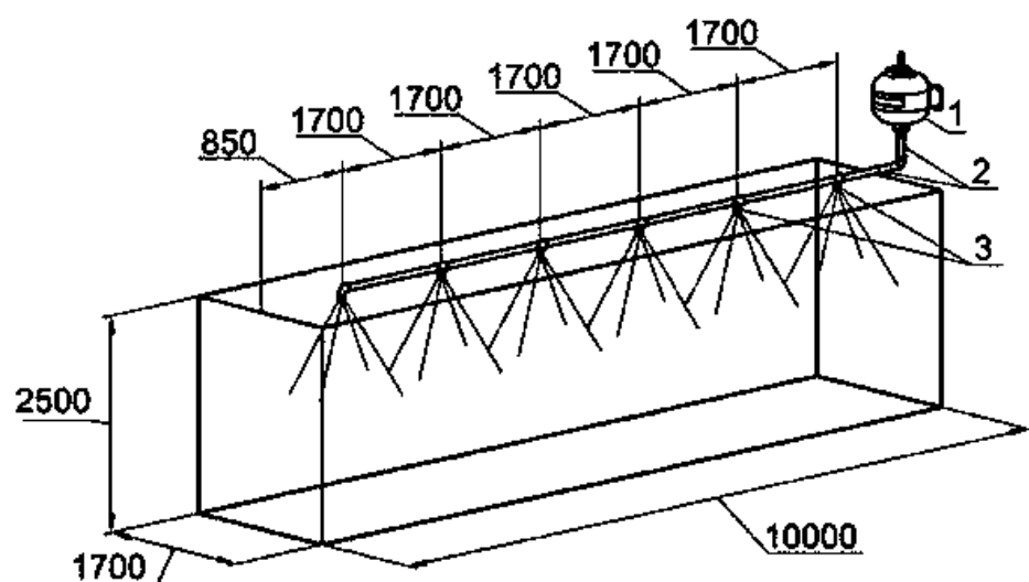
Рис.10. Монтажная схема распределительного трубопровода для модуля «Буран-15TPBTH2,5(Y1)», состоящего из одной ветви.
