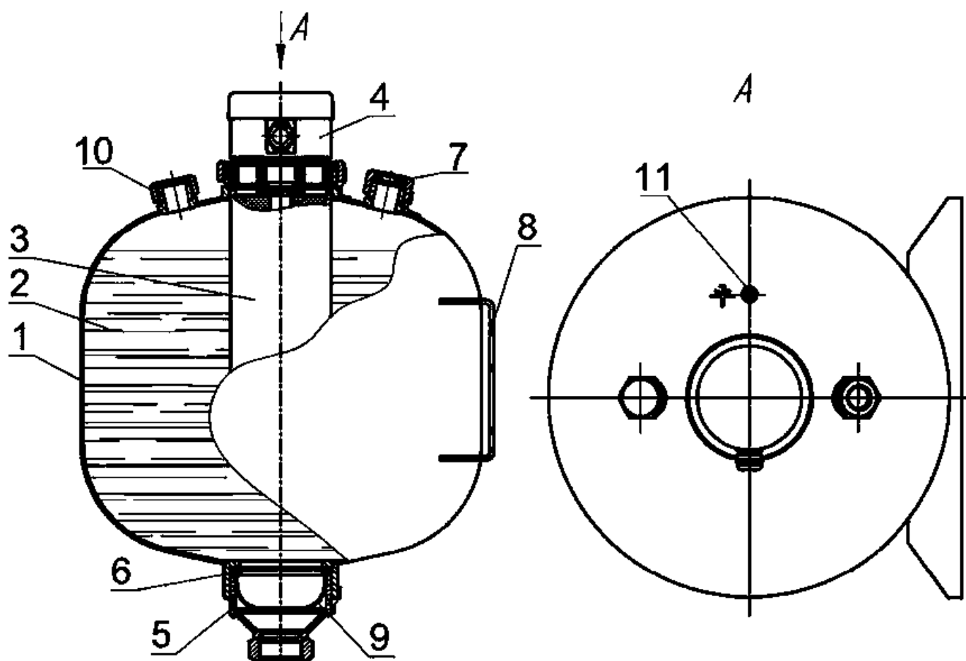
Рис.6. Устройство модуля пожаротушения тонкораспыленной водой «Буран-15ТРВТНТ(У1)».
