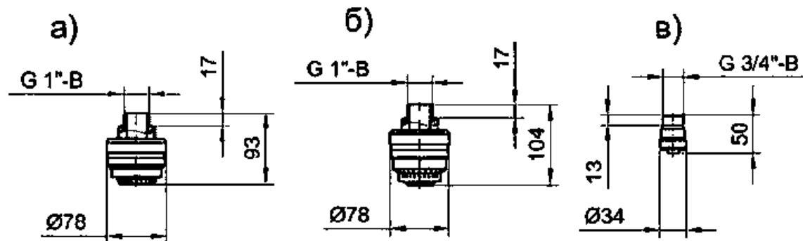
а) распылитель «ТРВ-6»; б) распылитель «ТРВ-4»; в) распылитель «ТРВ-2,5».
