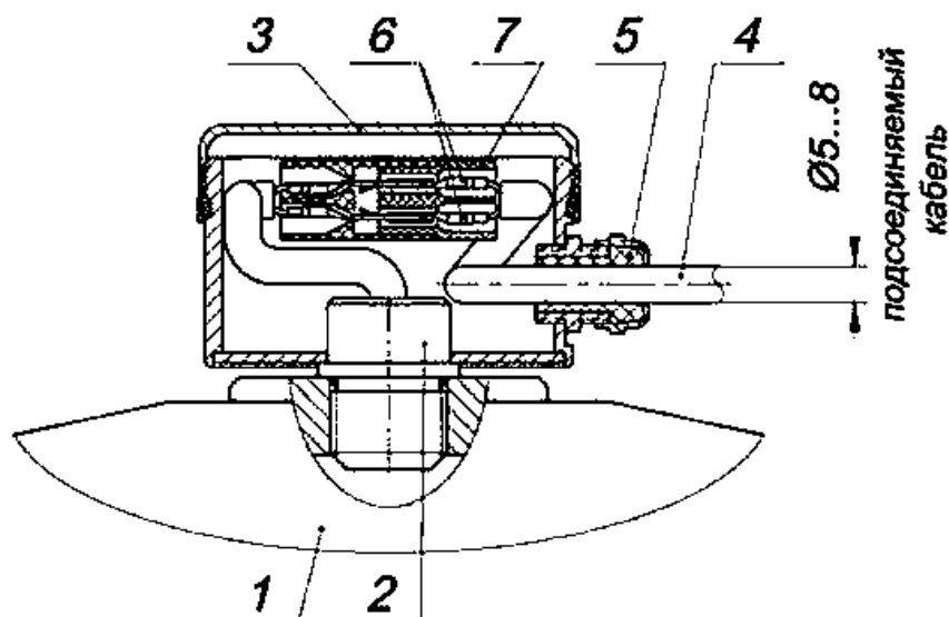
Рис.12 – Конструкция электровоспламенителя ЭСГ-0,5.
